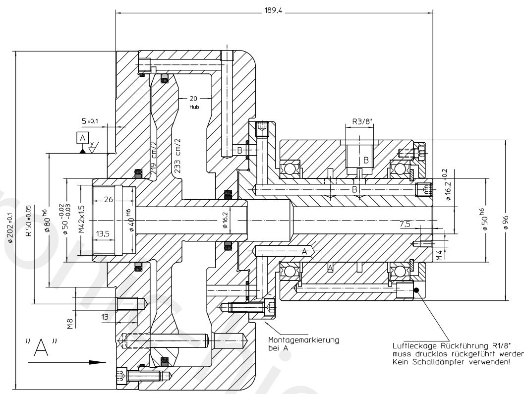
Ansicht "A"
